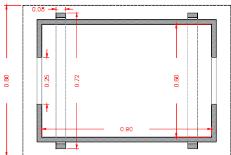
PLANTA
