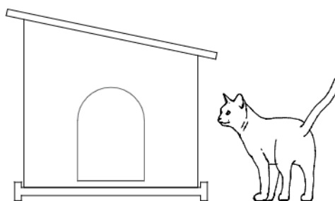
ALÇADO LATERAL
