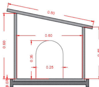
PERFIL TRANSVERSAL
